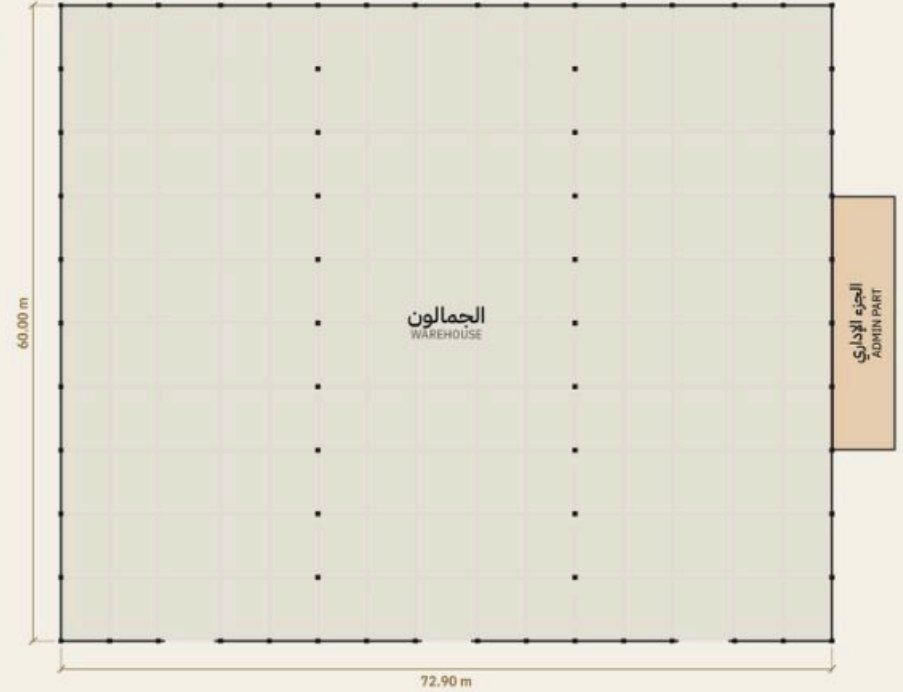
المسقط العام للجمالون
